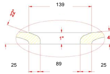
Détail évacuation
