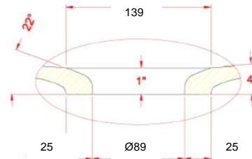
Détail évacuation
