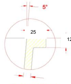
Détail paroi
