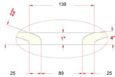
Détail évacuation
