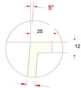
Détail paroi
